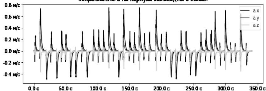
Компоненты линейного ускорения датчика, закрепленного на корпусе самоходного шасси
