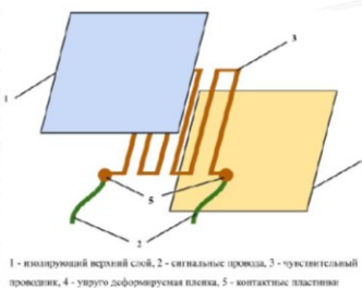
Рисунок 8 - тензорезистор
