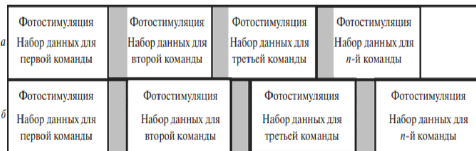
Рис. 1. Схема времени обработки ЭЭГ для выделения SSVEP.
