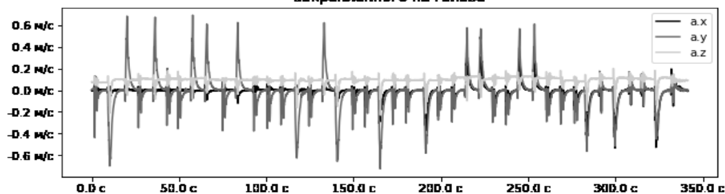
Компоненты линейного ускорения датчика, закрепленного на голове
