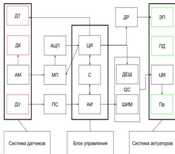
Блок-схема системы обратной связи
