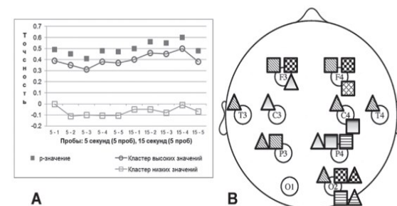
Рисунок 1. А - кластеры высоких и низких значений при шкалировании коротких интервалов времени. * - p < 0,001 . В - различия СПМ между кластерами: ■ - проба 5 секунд, тета-ритм; ▲ - проба 15 секунд, тета-ритм; ▨ - проба 5 секунд, альфа-ритм; ▩ - проба 15 секунд, альфа-ритм; ▪ - проба 5 секунд, бета-нижний; ▴ - проба 15 секунд, бета-нижний; ▸ - проба 5 секунд, бета-верхний; ▹ - проба 15 секунд, бета-верхний. Различия достоверны: p < 0,01 .
