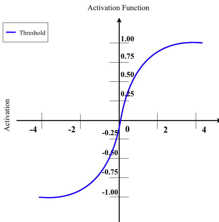
Рисунок 12 – Гиперболический тангенс
